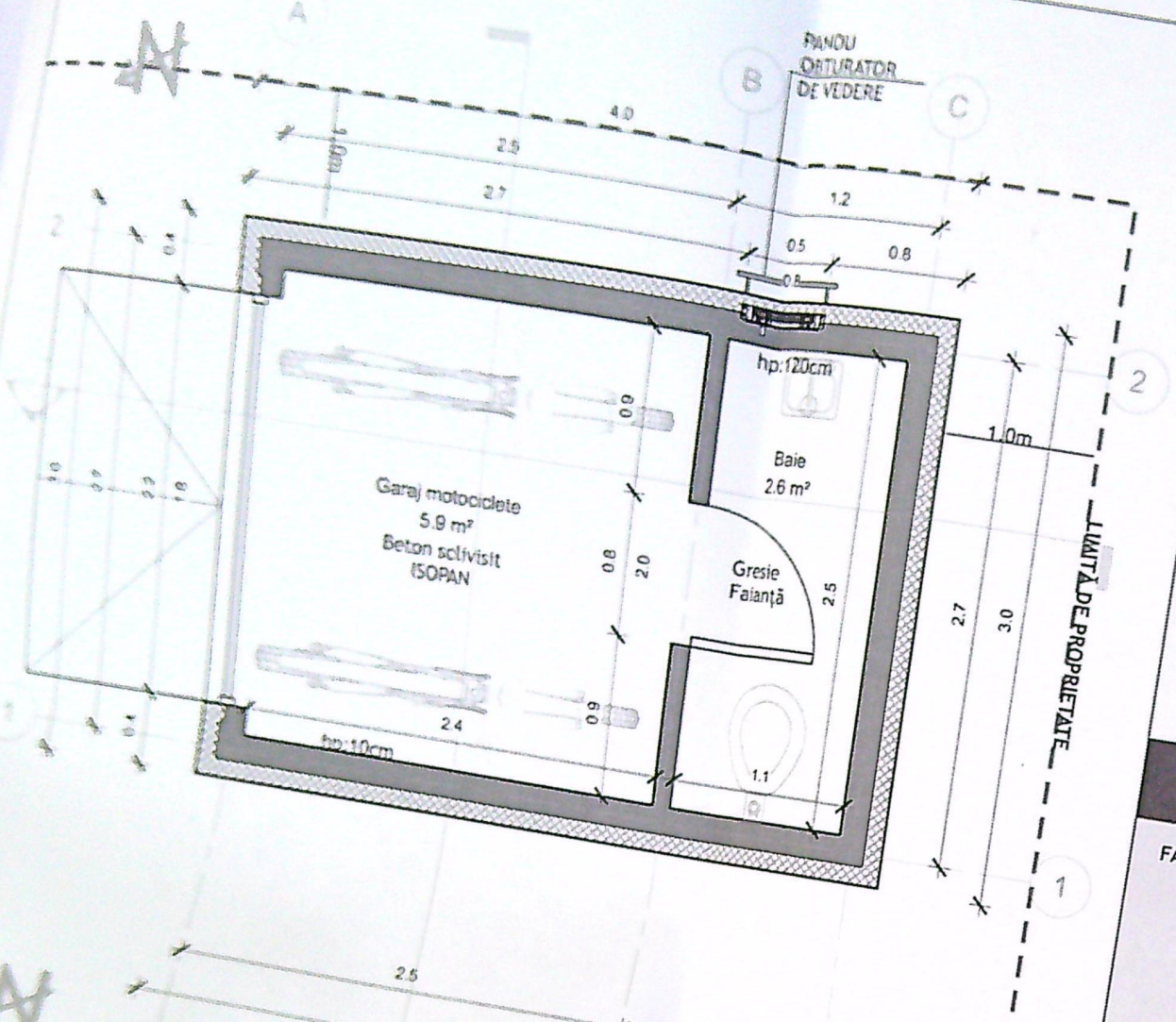
SECȚIUNE A-A' SC:1/50
